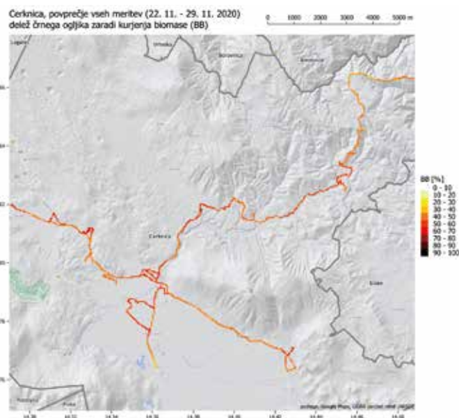
Povprečni prispevek kurjenja biomase h koncentracijam BC za vse meritve v obdobju od 22. do 29. novembra 2020
