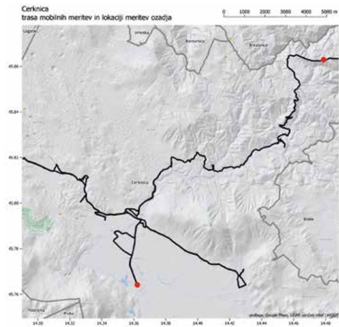
Trasa mobilnih meritev v občini Cerknica in lokaciji meritev ozadja
