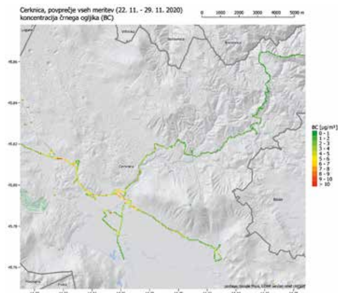
Karta povprečnih koncentracij črnega ogljika z upoštevanjem vseh opravljenih meritev od 22. do 29. novembra 2020
